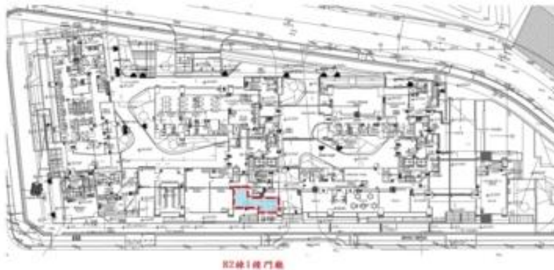
附件四 1樓配置圖
