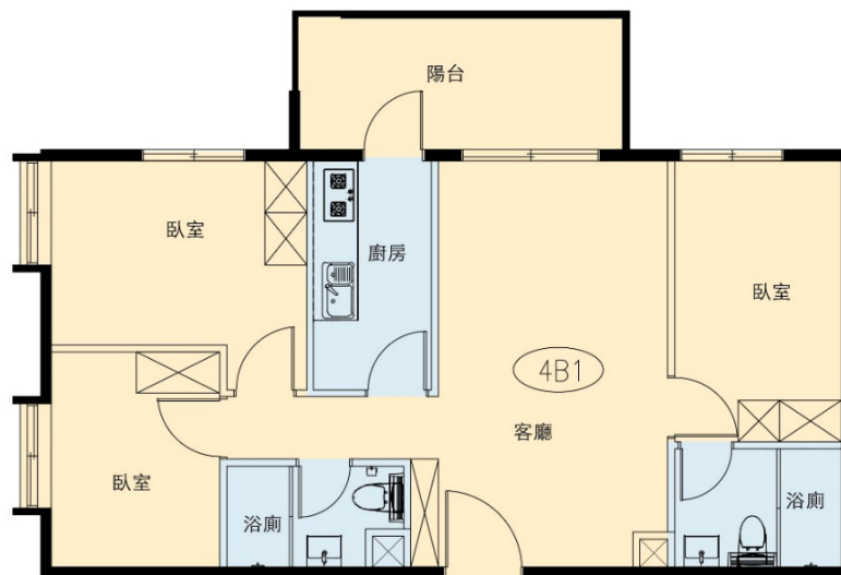
圖 7_興隆社會住宅 I 區三房型配置表
