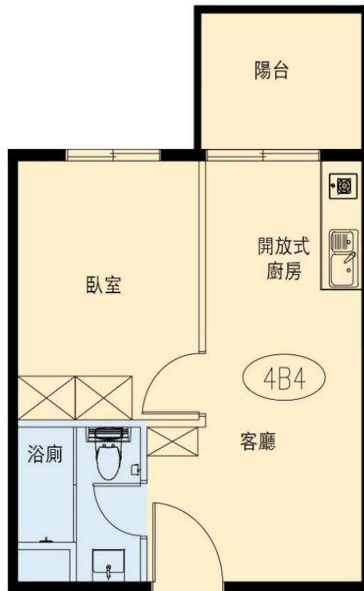
圖 5_興隆社會住宅 I 區一房型配置表
