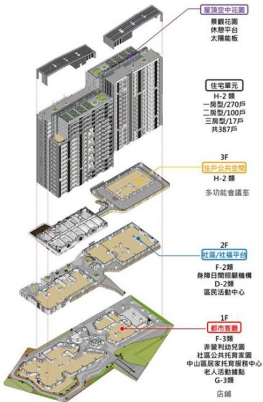
圖 3_錦州社宅各樓層空間示意圖
