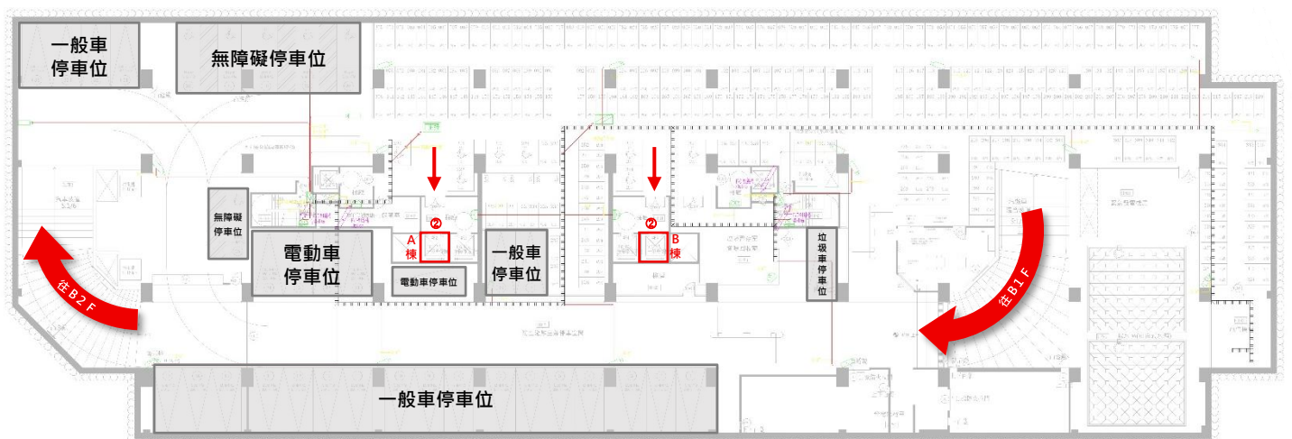
圖一 地下一層(B1F)平面圖
