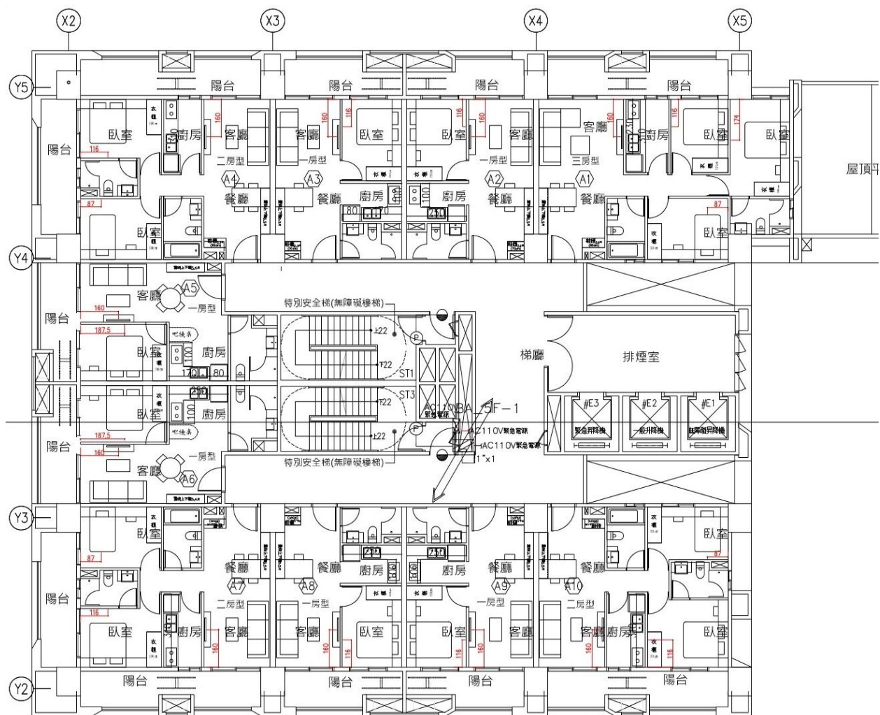
一般房型電視補強板配置平面圖 (A 棟 5F~20F)
