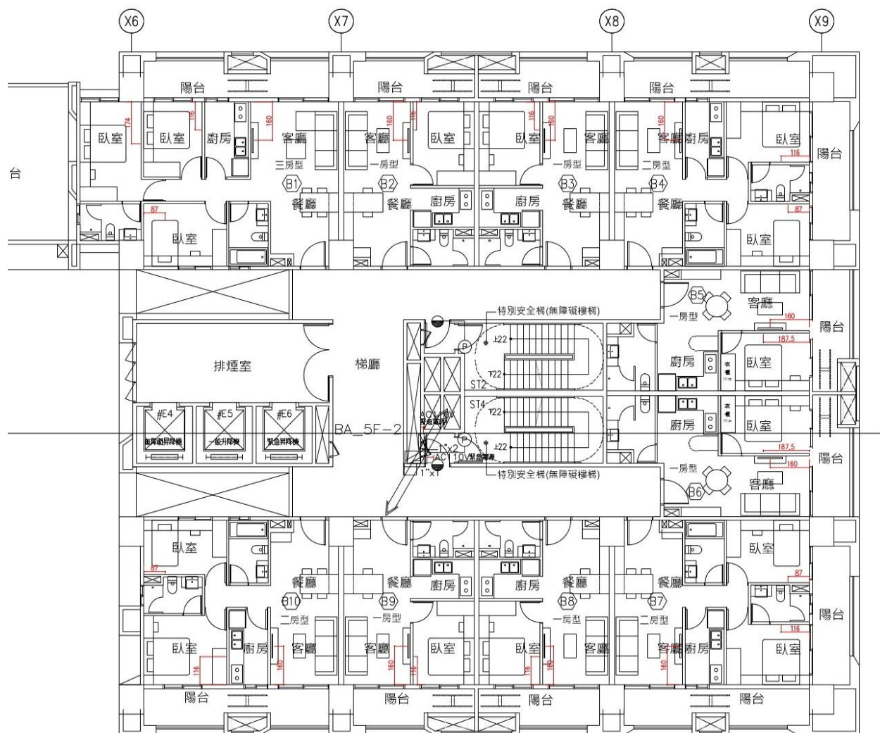
一般房型電視補強板配置平面圖 (B棟 5F~20F)
