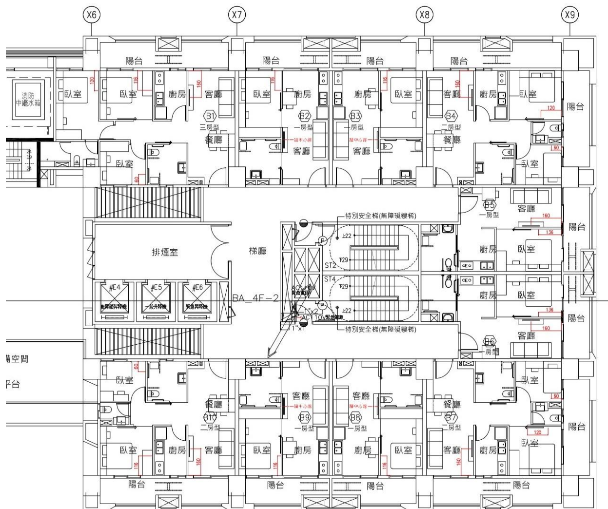
無障礙房型電視補強板配置平面圖 (B棟 4F)
