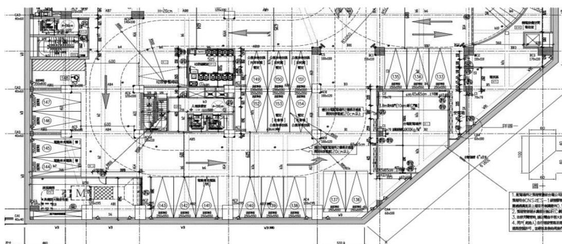
圖一 地下一層(B1F)平面圖
