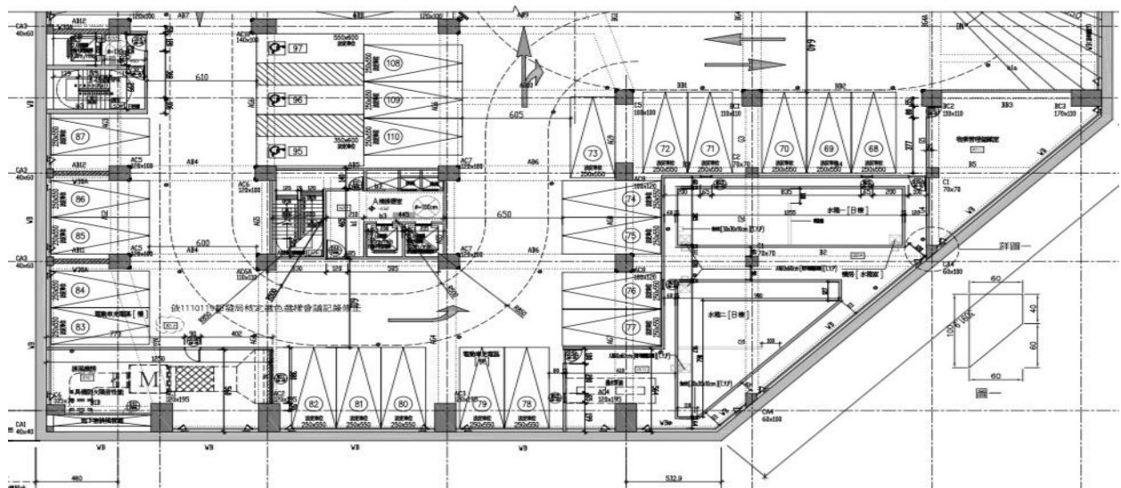
圖二 地下二層(B2F)平面圖
